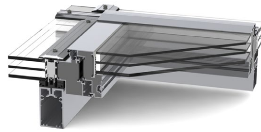
Variante 2 de notre vantail d'aération LAMILUX Ventilation Flap PR60 Avec une surface d'écoulement plane et lisse pour des inclinaisons de toit de 2° à 75°
