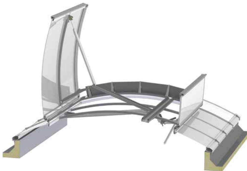
SYSTÈME CI EXUTOIRE DE FUMÉES TYPE B EN TANT QUE CLAPET DOUBLE ASYMÉTRIQUE
